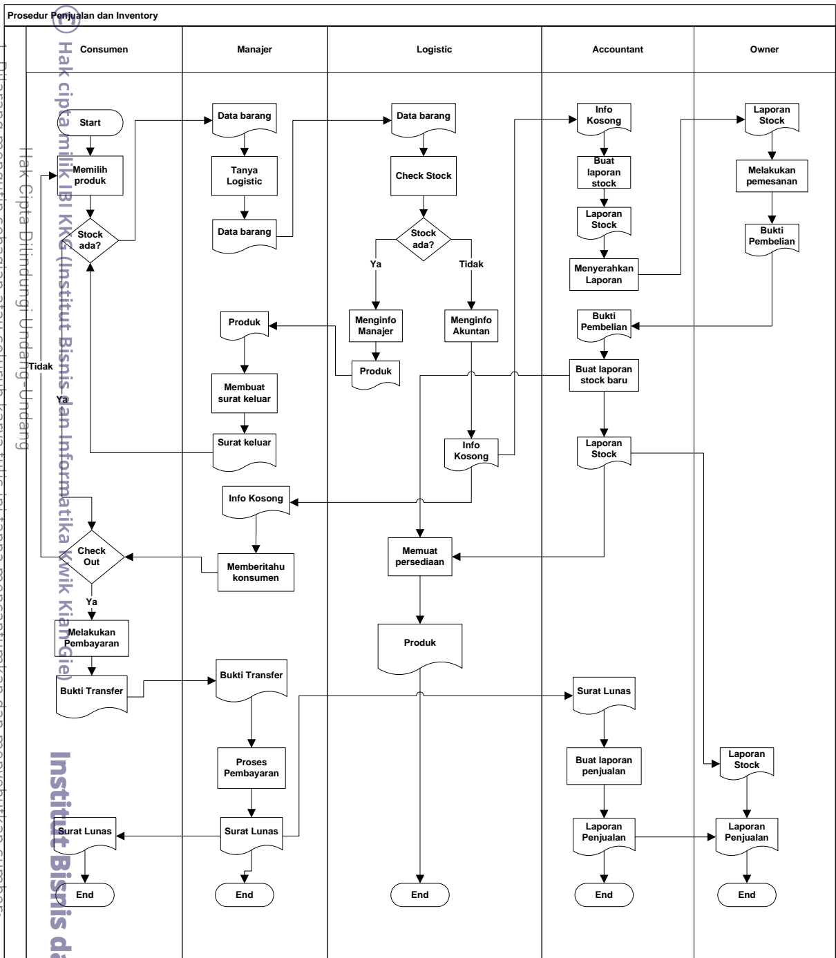
Gambar 3.2 Flowchart Prosedur Penjualan dan Inventory
