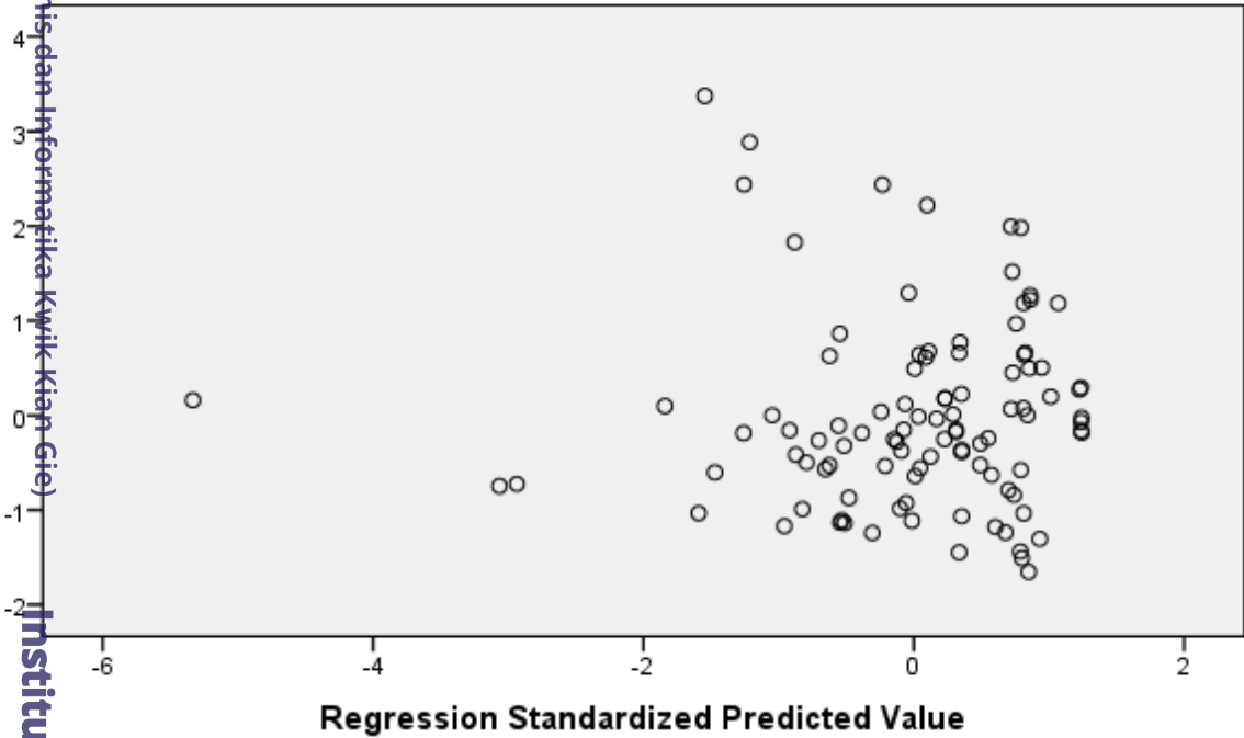
Scatterplot Dependent Variable: DER
