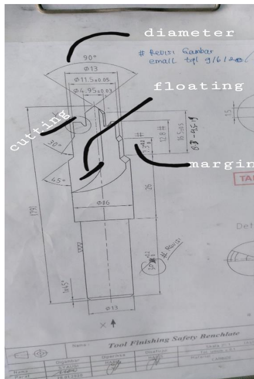
Gambar 5. 2 Lembar Sketsa Produk Custom
