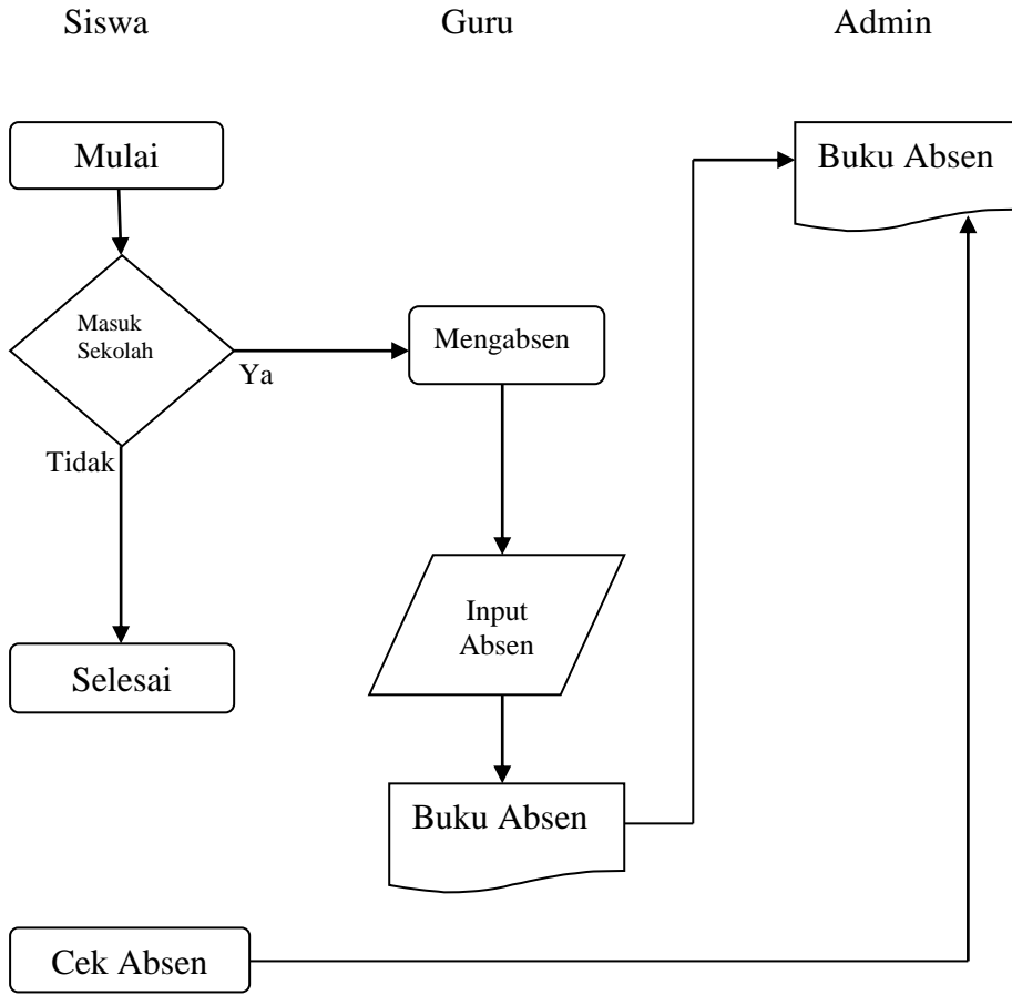
Gambar 3.2 Proses Sistem Absensi Siswa
