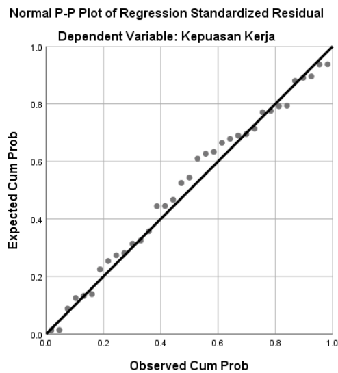
Output Uji Normalitas Probability Sebelum di Lakukan Eliminasi Data
