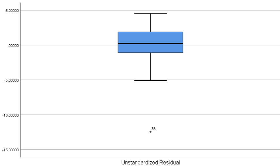
Output Box Plot Sebelum Dilakukan Eliminasi Data No Responden 33
