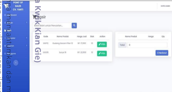
Gambar 12. Halaman Kasir
