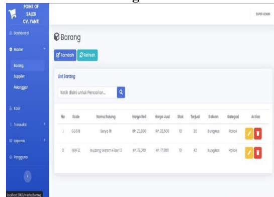
Gambar 9. Halaman Barang
