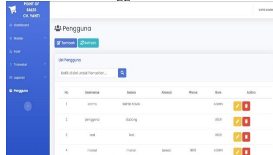
Gambar 15. Halaman Pengguna
