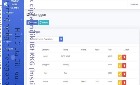
Gambar 11. Halaman Pelanggan
