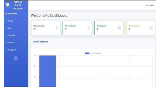
Gambar 8. Halaman Utama
