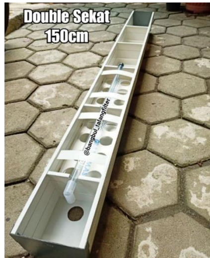
Gambar 5.8 Talang Air 150 cm
